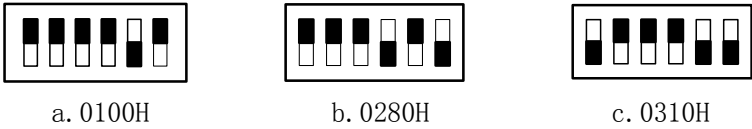
图 3 I / O 基地址选择举例
