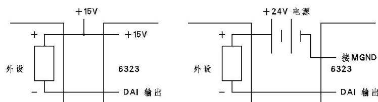
a. 使用为本卡提供的+15V 电源 b. 使用机外+24V 电源
