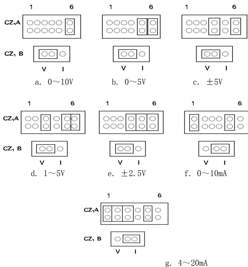
图 4 D / A 输出量程及方式选择
