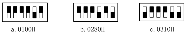
图 3 I / O 基地址选择举例
