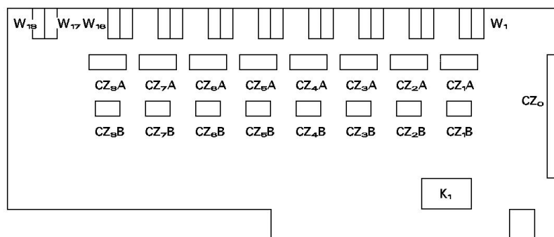
图2 主要可调整元件位置图
