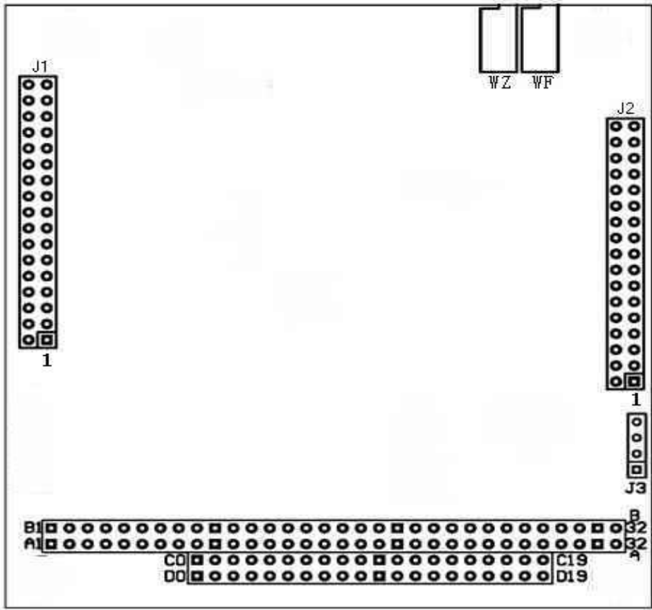
3. 1. 1 模拟输入管脚图——J1
