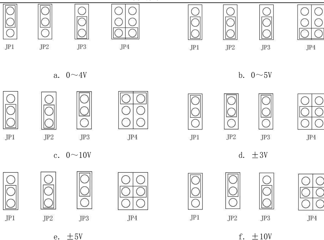
图2 A/D 量程选择
